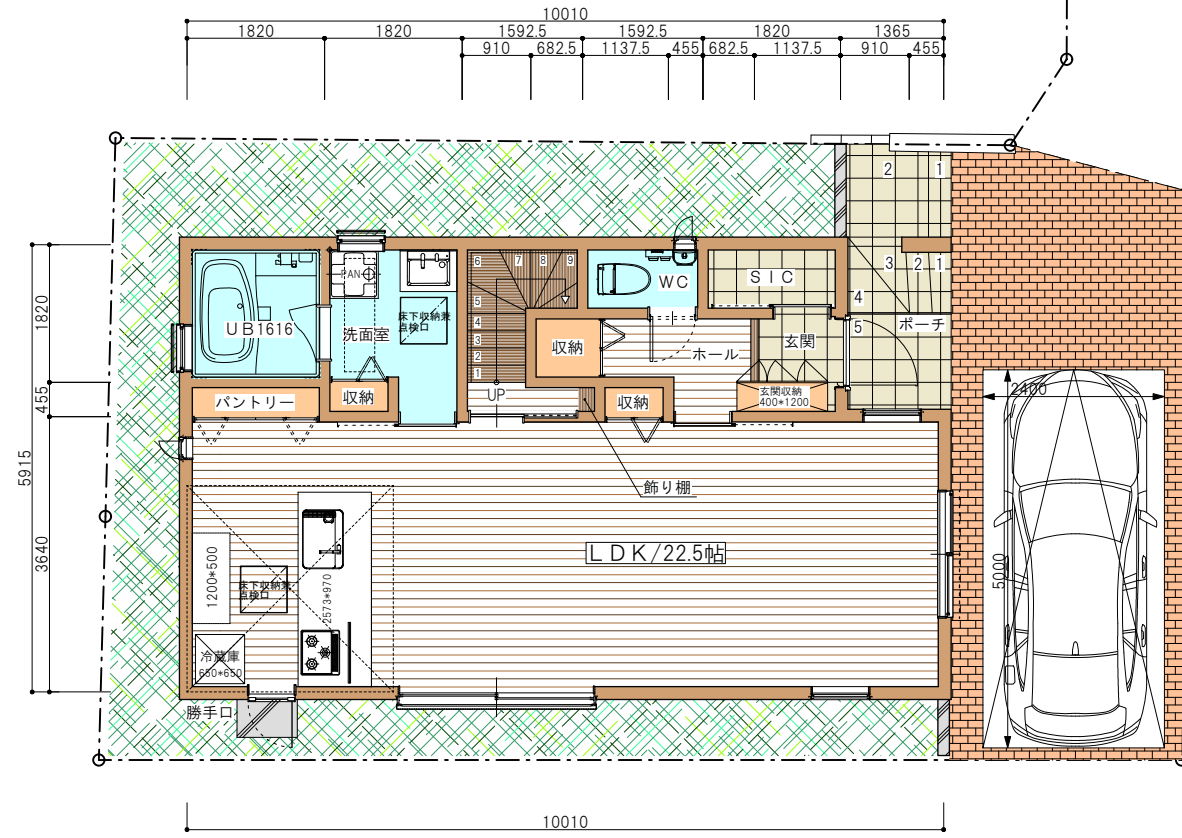
1階平面図
