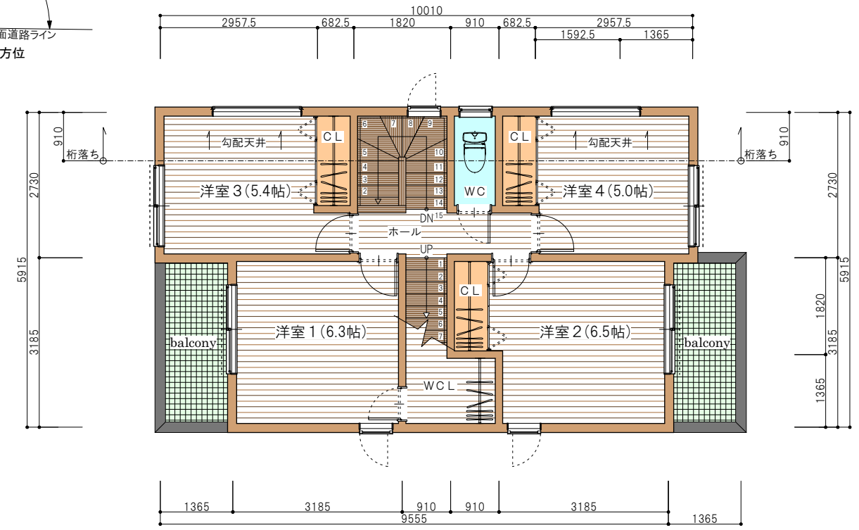
2階平面図
